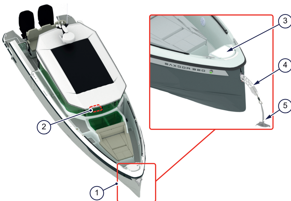
Figur 5.8 - Ankarsystem
