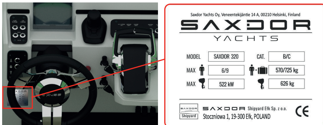
Figur 4.20 - Tillverkarskylt
