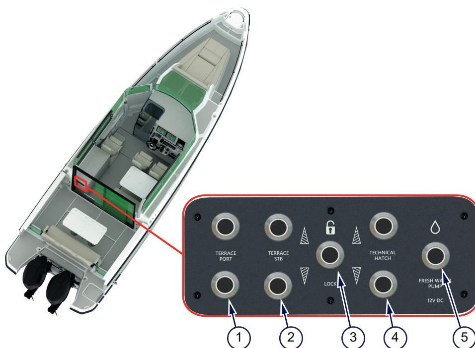
Figur 4.13 - Terrasskontrollpanel
