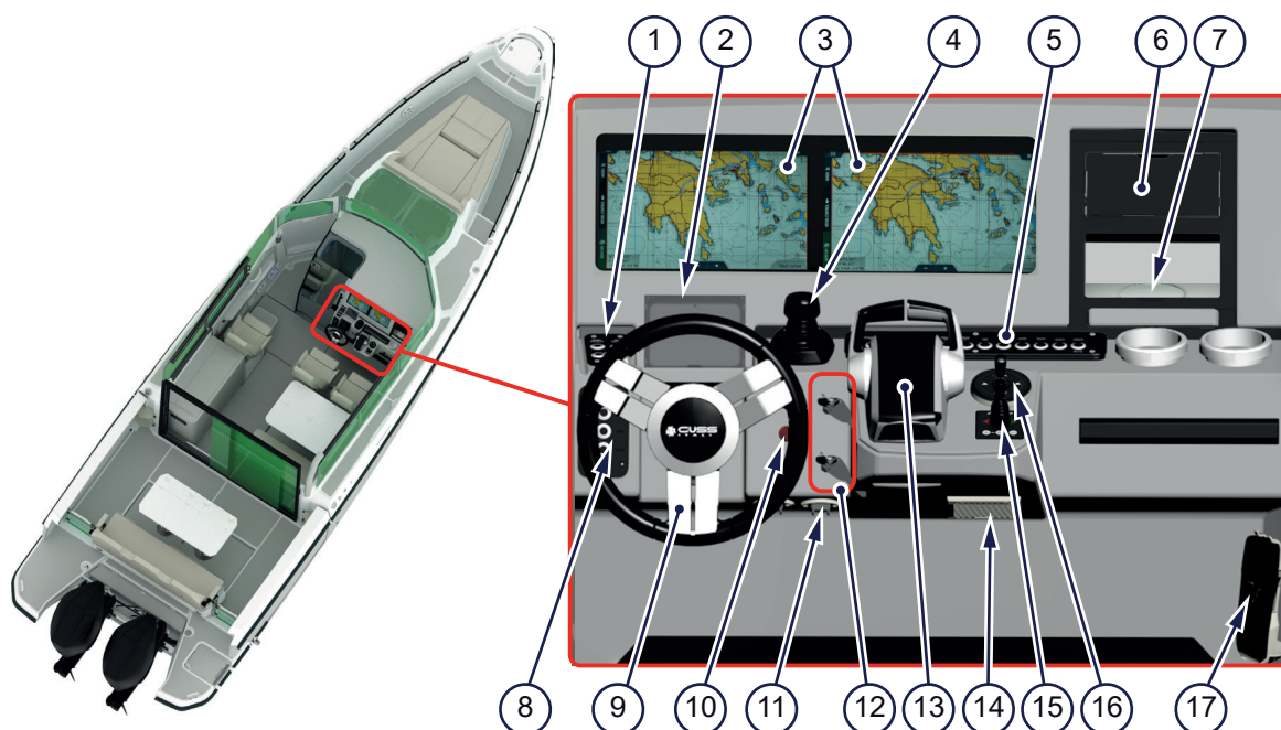
Figur 4.8 - Förarplatsens reglage
