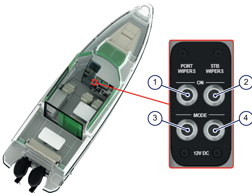
Figur 4.11 - Torkarkontrollpanel
