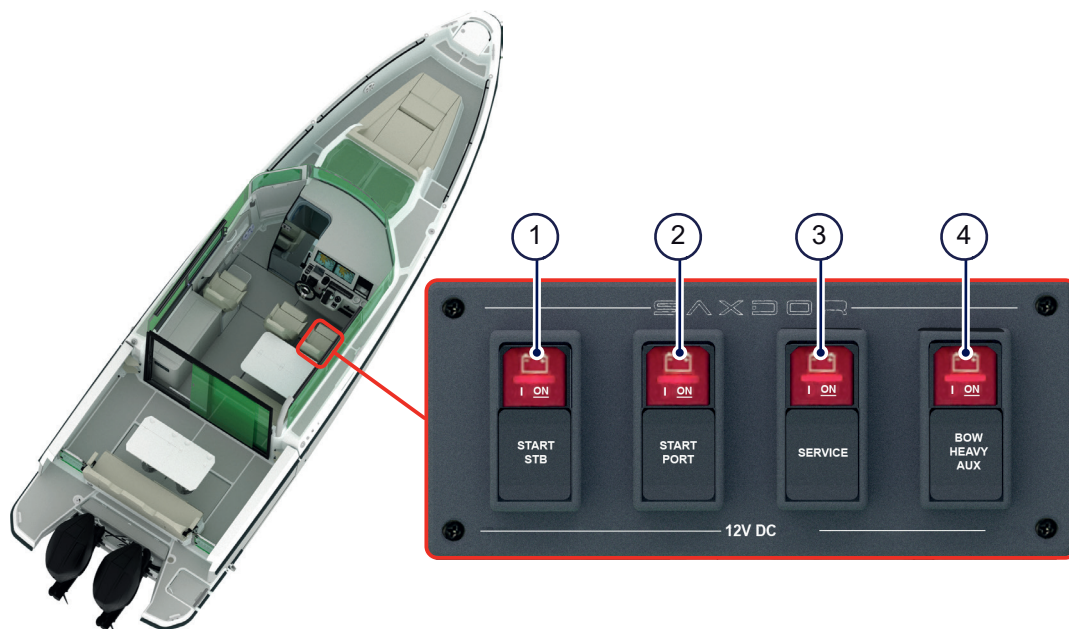
Figur 4.16 - Batterikontrollpanel
