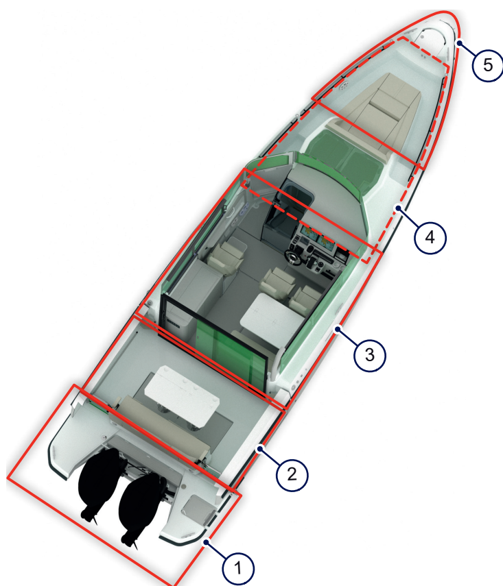
Figur 4.1 - Allmän båtlayout
