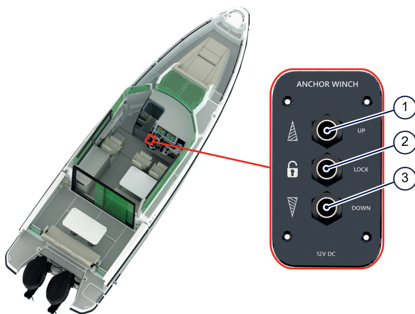
Figur 4.10 - Ankarspelets kontrollpanel
