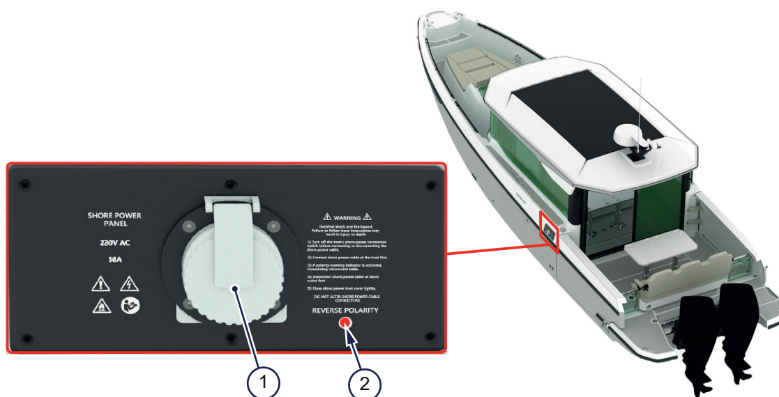
Figur 4.17 - Landströmspanel
