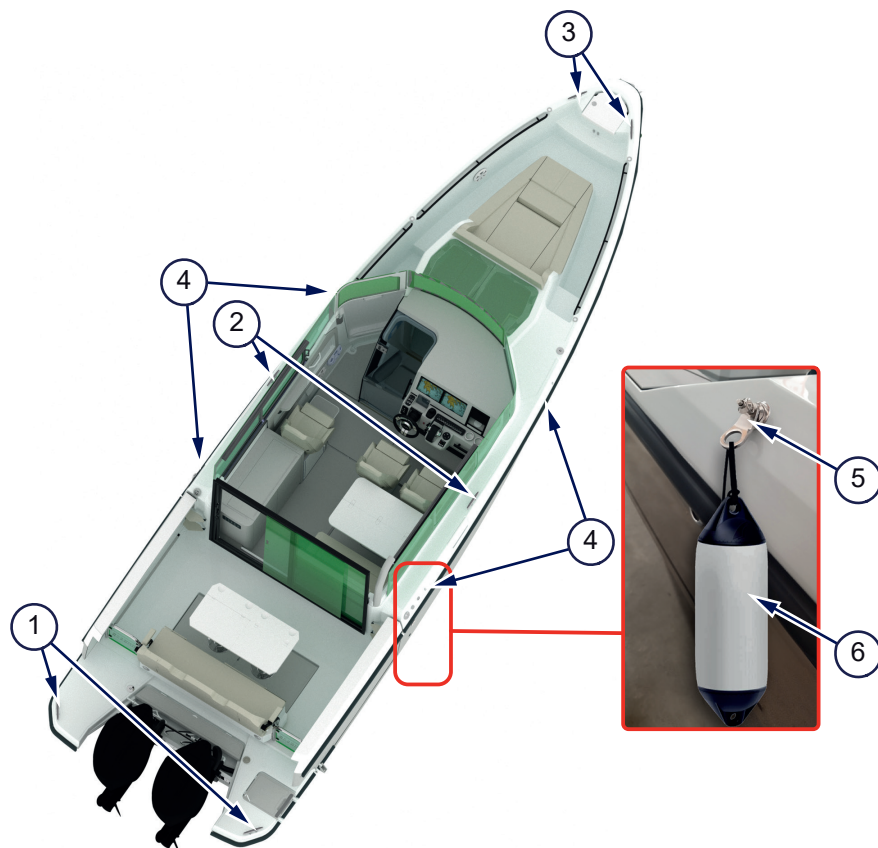
Figur 4.24 - Fästpunkter
