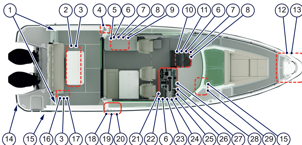
Figur 4.23 - Säkerhetsmärkningens placering på din båt
