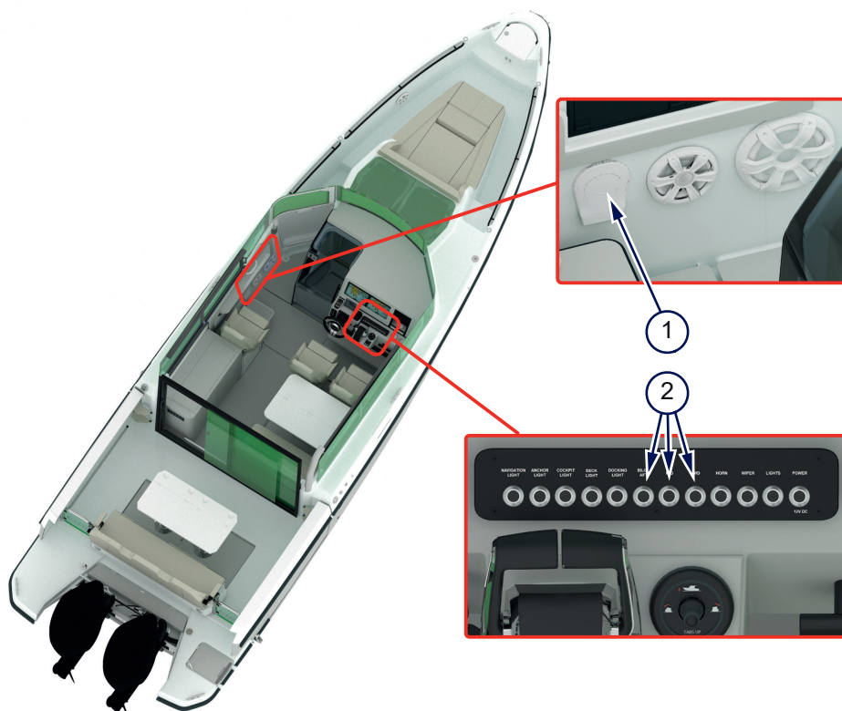
Figur 5.5 - Manuell läns pump och de automatiska läns pumparnas reglage
