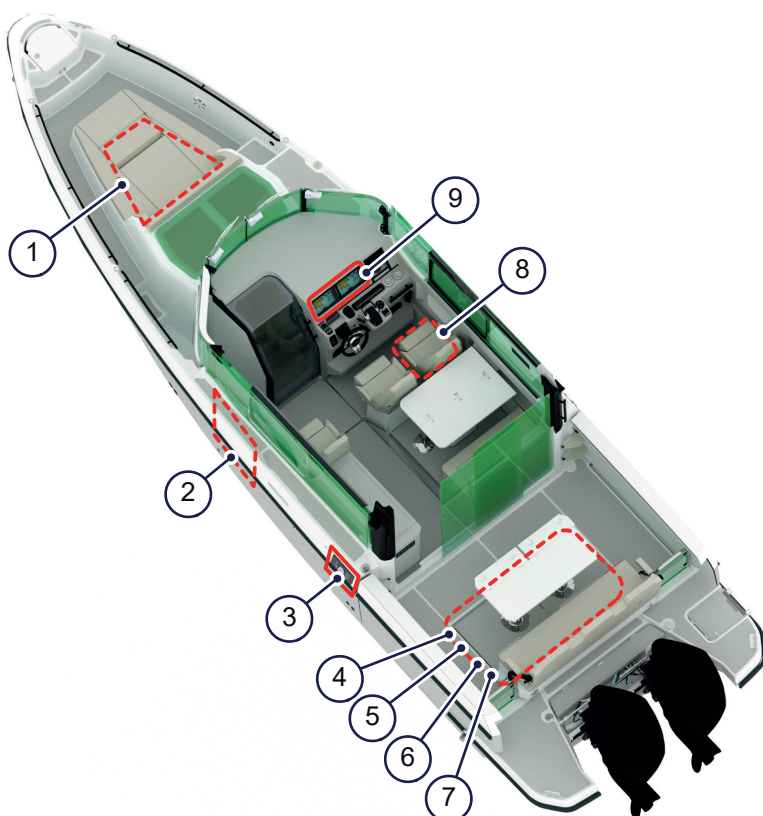
Figur 5.1 - Elsystem
