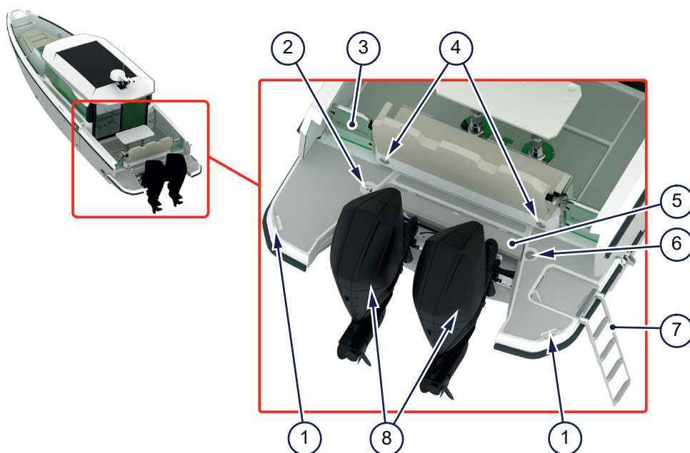
Figur 4.6 - Badplattform
